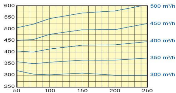
Рисунок 20 — D250, диапазон 500–800 м³/ч
